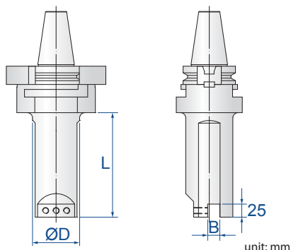
ID Tool Holder (IDF)
